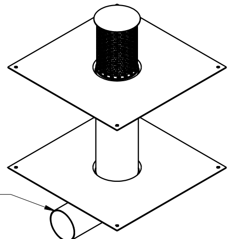
Variante mit Abgang horizontal
