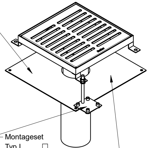
Klebeblech aufgeraut
