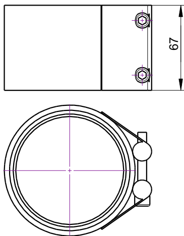
Bride Nr. 116742 \varnothing 125/131 mm
