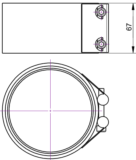
Bride Nr. 116667 \varnothing 110/114.3 mm
