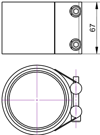
Bride Nr. 116829 \varnothing 75/76.1 mm
