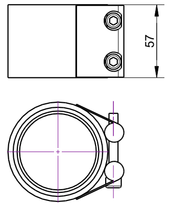
Bride Nr. 116821 \varnothing 63/63.5 mm
