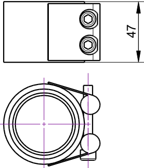
Bride Nr. 116815 \varnothing 48/50 mm
