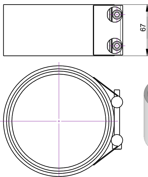
Bride Nr. 116742 \varnothing 125/131 mm
