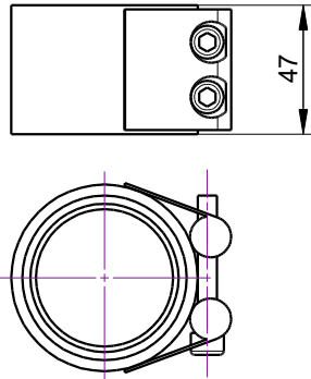
Bride Nr. 116826 \varnothing 54/56 mm
