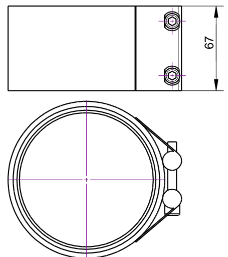
Bride Nr. 116763 \varnothing 110 mm
